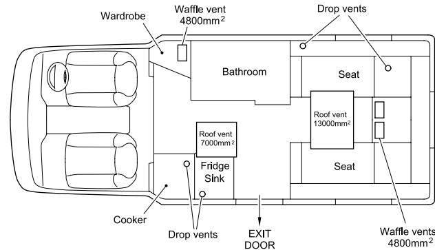
Ventilation - Roadstar EL
